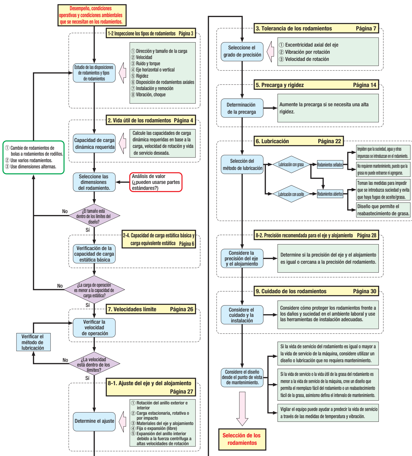
● Figura 1.1 Procedimiento para seleccionar los rodamientos
