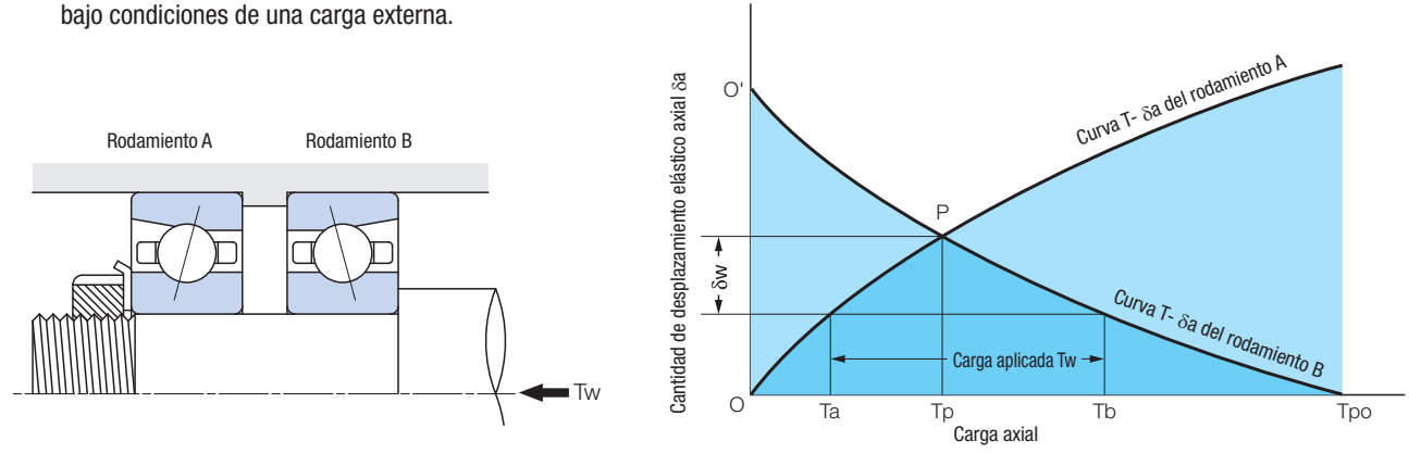
● Figura 5.3 Precarga de posición fija
