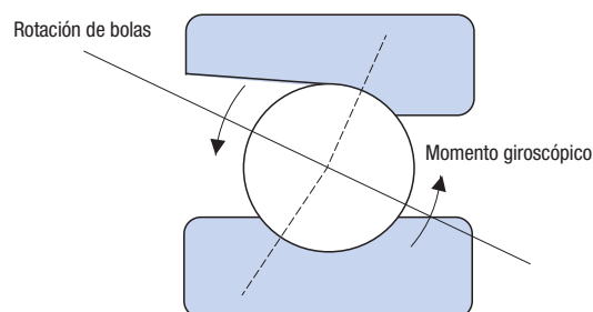
● Figura 5.1 Momento giroscópico
