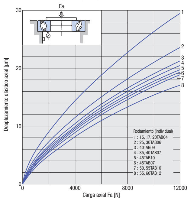
Carga axial y desplazamiento axial
