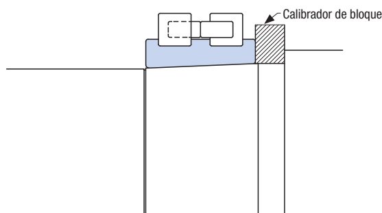
● Figura 9.10 Medición de la dimensión del ancho temporal del espaciador
