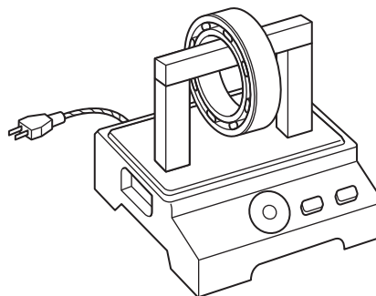
● Figura 9.2 Calentador de inducción
